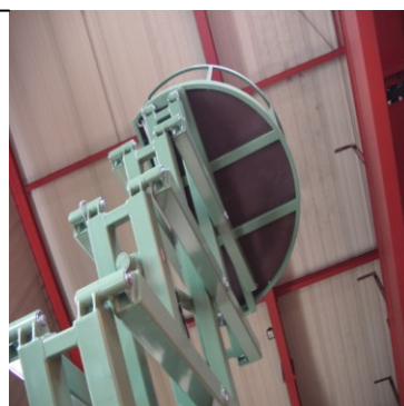
工作平台为半圆形的剪叉式升降台，用于航空火箭研究制造
