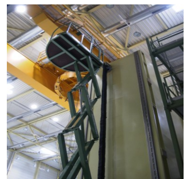
工作平台为半圆形的剪叉式升降台，用于航空火箭研究制造
